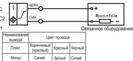
Схема подключения к оборудованию
