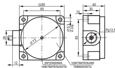
Габаритный чертеж
